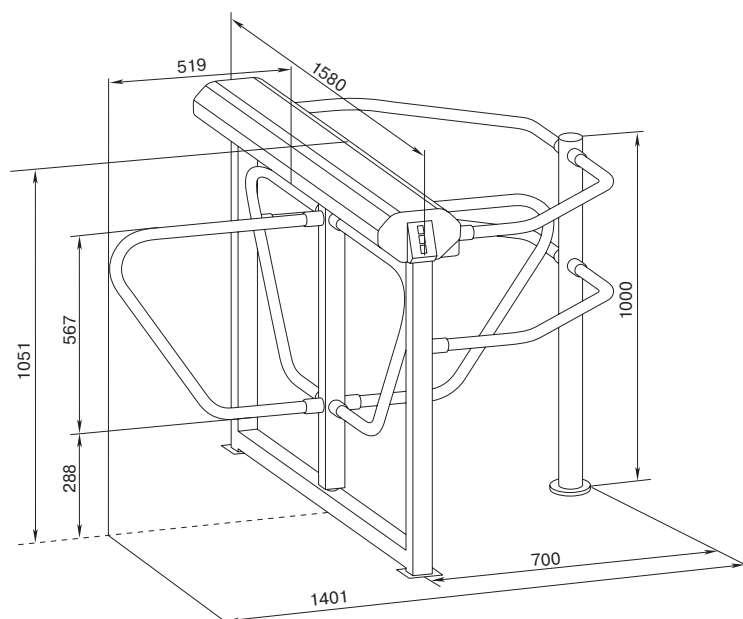
Габаритные размеры
