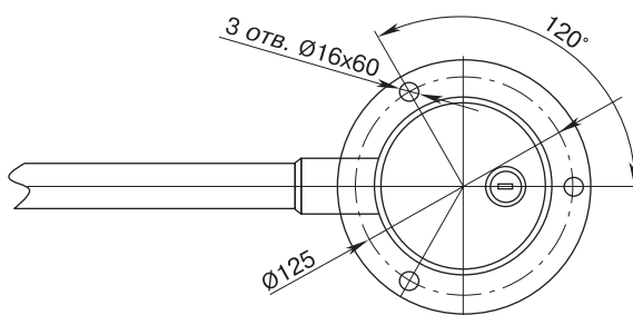
Схема разметки отверстий для калитки
