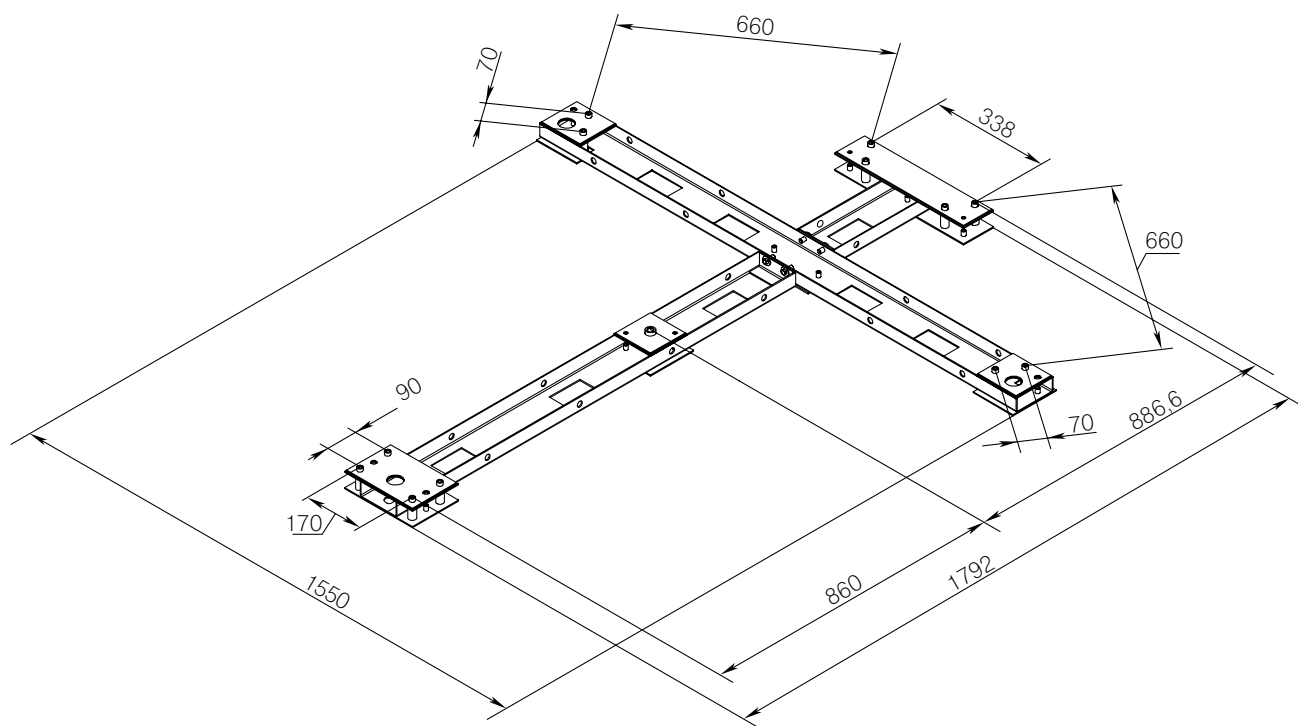
Установка рамы
