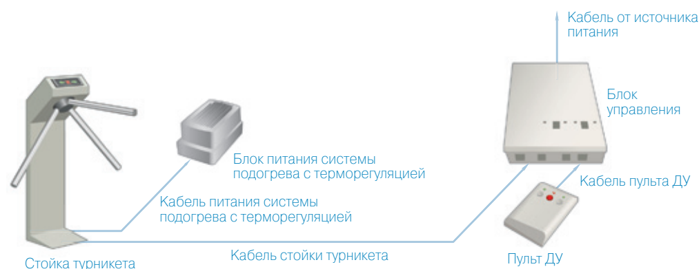
Схема подключения турникета PERCo-T-04W-24.
