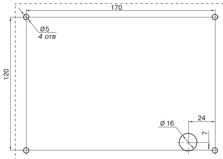
Разметка отверстий для установки контроллера PERCo-CR01
