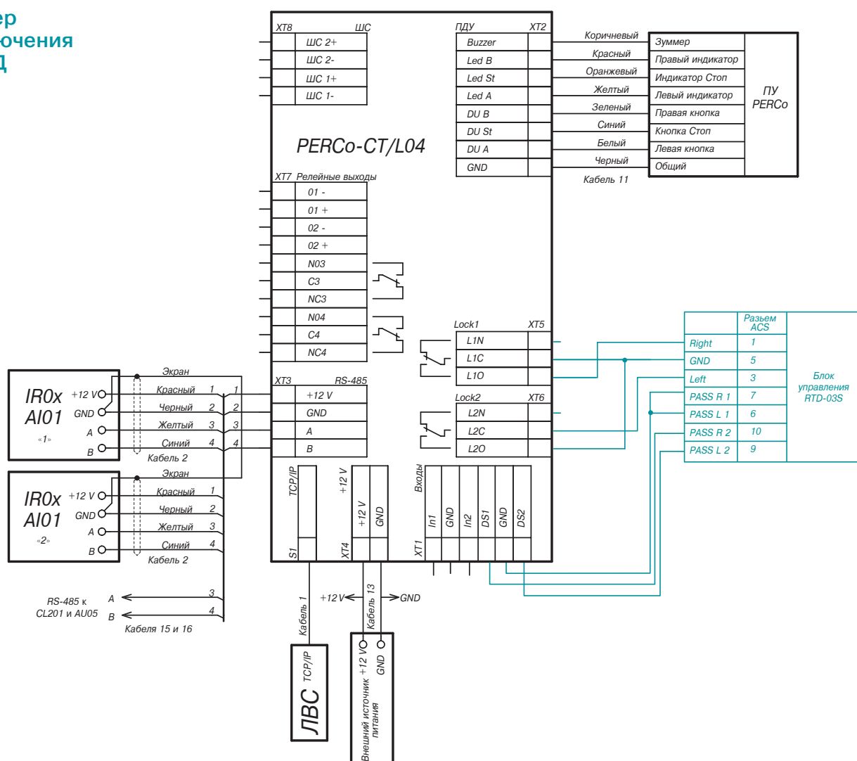
Пример схемы подключения турникета к контроллеру СКУД (на примере контроллера PERCo-CT/L04)
