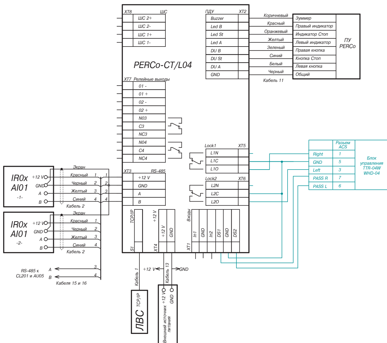
Пример схемы подключения калитки к контроллеру СКУД
