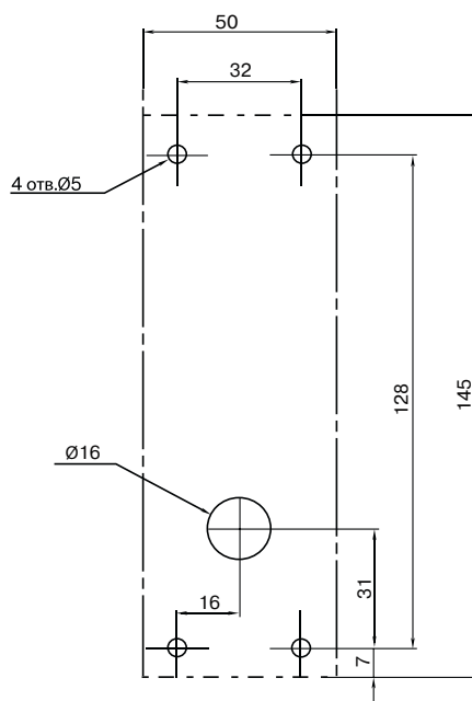
Разметка отверстий для установки блока индикации
