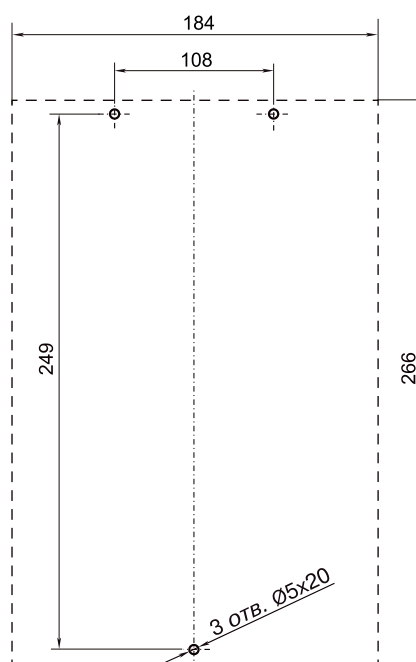
Схема разметки отверстий для установки блока управления
