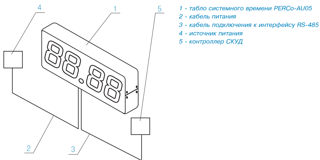
Схема подключения
