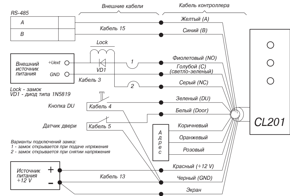
Схема подключений контроллера PERCo CL201
