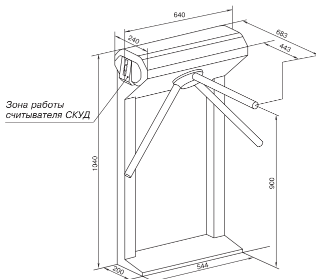
Габаритные размеры
