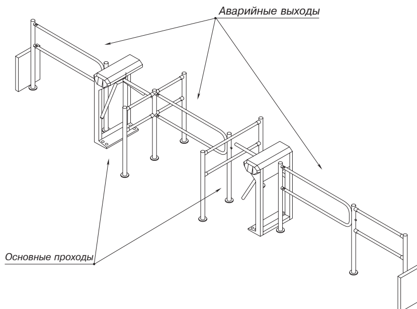
Пример проекта проходной
