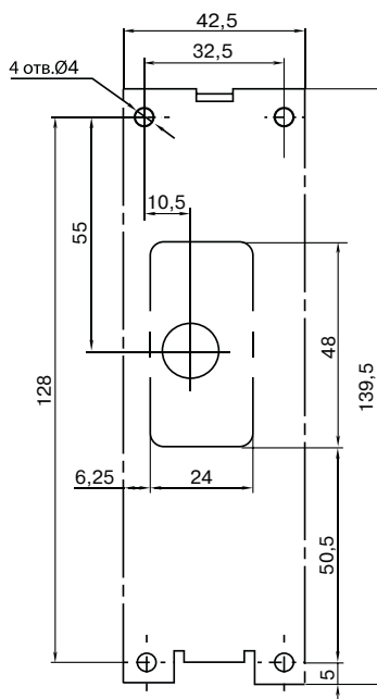
Разметка отверстий для установки контроллера PERCo-CL05
