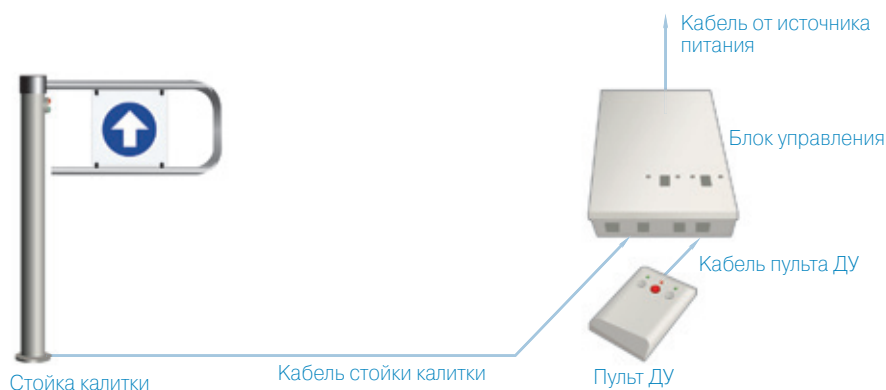
Схема подключения калитки PERCo-WHD-04
