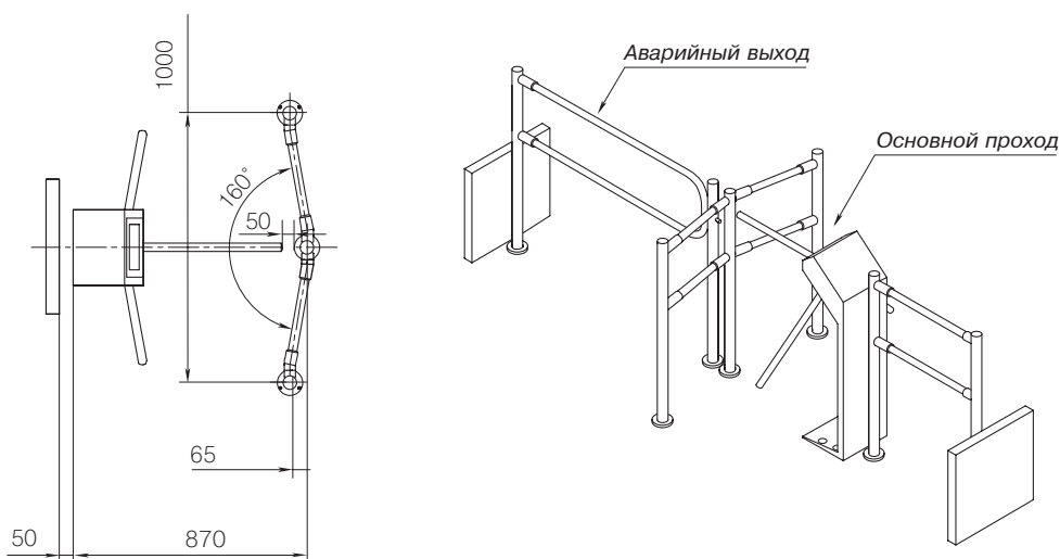
Вид турникета сверху
