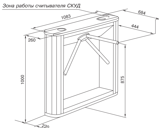
Габаритные размеры
