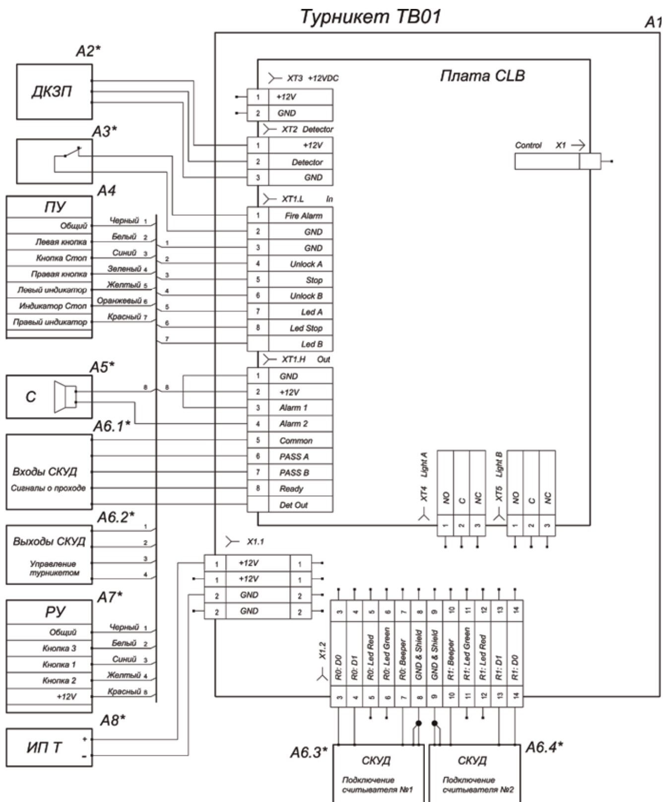
Схема внешних подключений турникета PERCo-TB01
