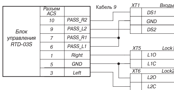
Схема подключения полуростового роторного турникета PERCo-RTD-03S
